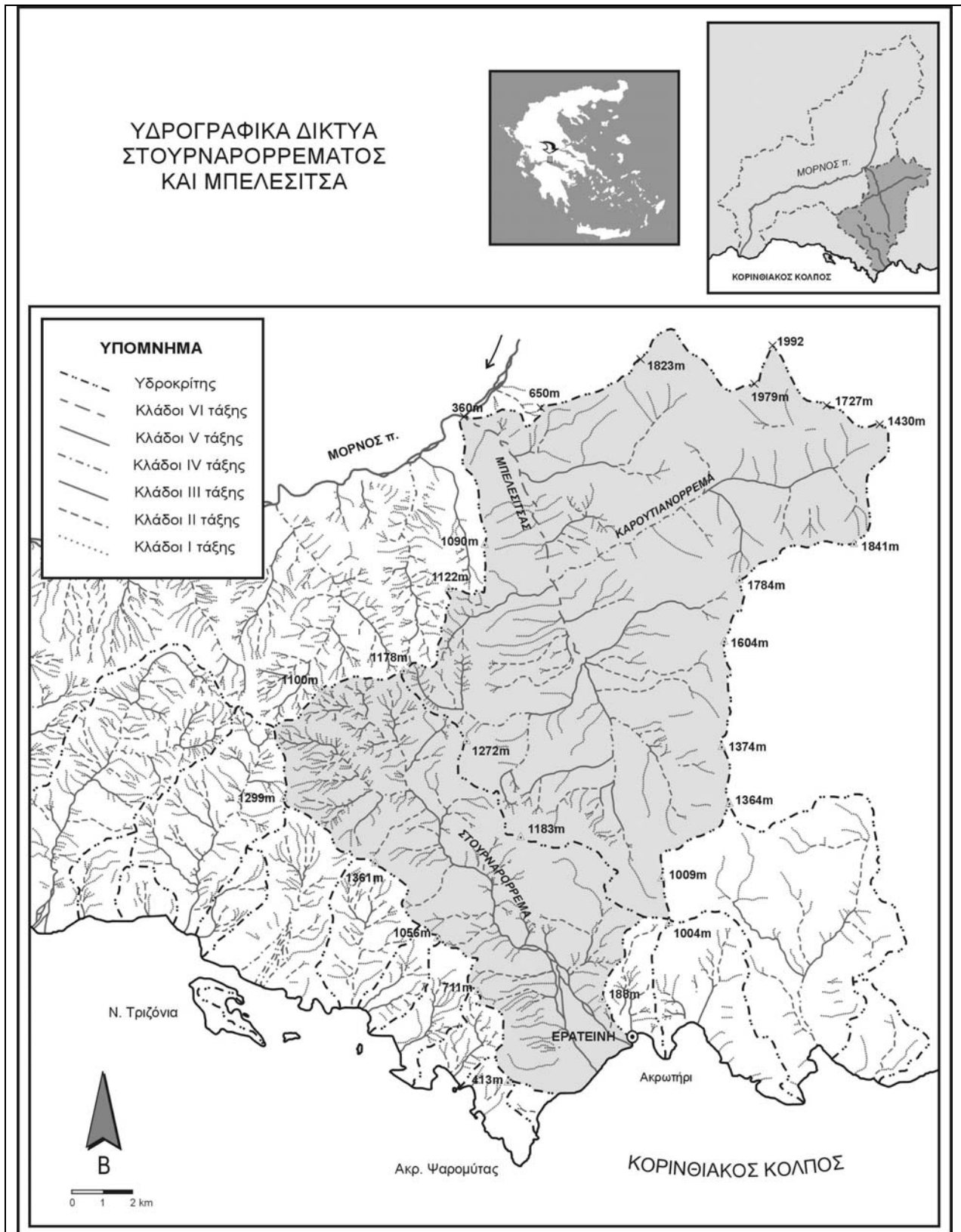
Εικ. 1 : Το υδρογραφικό δίκτυο της ευρύτερης περιοχής της Ερατεινής, όπου διακρίνεται η παράλληλη ανάπτυξη των λεκανών του Στουρναρορρέματος και του Μπελεσίτσα και η ταυτόχρονη αντίθετη αποστράγγισή τους.
